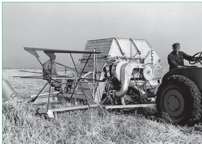
Перший причіпний комбайн CLAAS MDB – «Mahdreschbinder»: «Косить-обмолочує-зв'язує» (1936)
